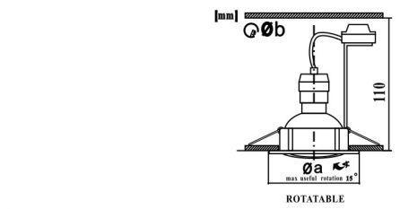
ROTATABLE
